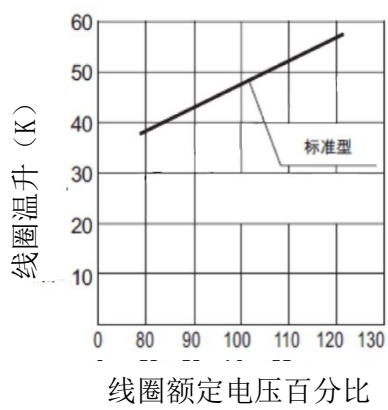
温升曲线
