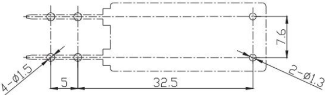
安装孔位图 (底视图)
