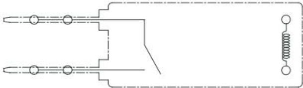
1A 接线图 (底视图)
