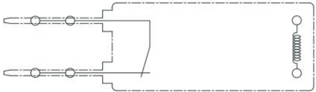
1B 接线图 (底视图)
