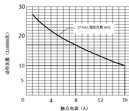
寿命曲线
