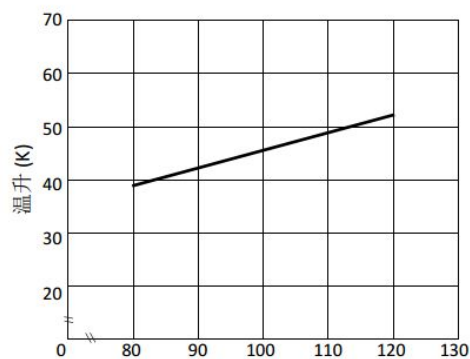
线圈温升
