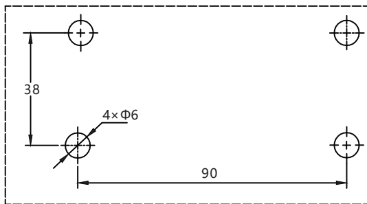
安装尺寸
