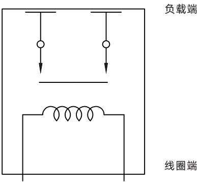
原理图
