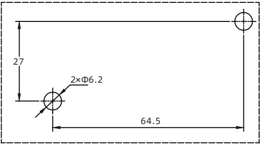
安装尺寸
