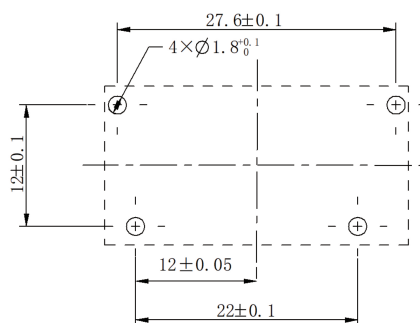
安装孔位图 (底视图)
