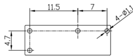
安装孔尺寸图 (底视图)
