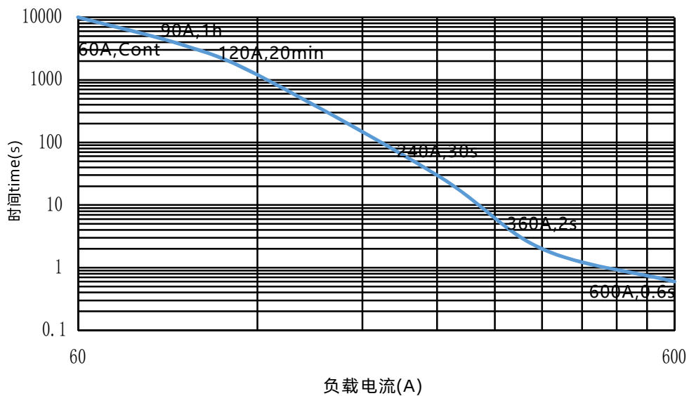
耐受能力曲线图
