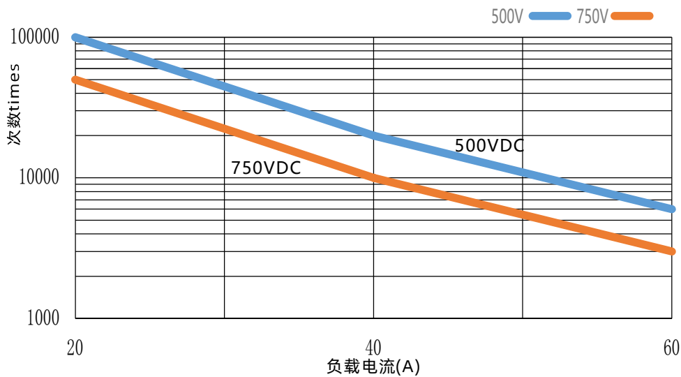
带载切换寿命曲线图
