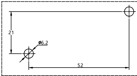
安装尺寸
