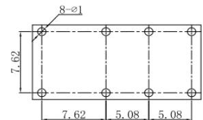
安装孔尺寸图 (底视图)
