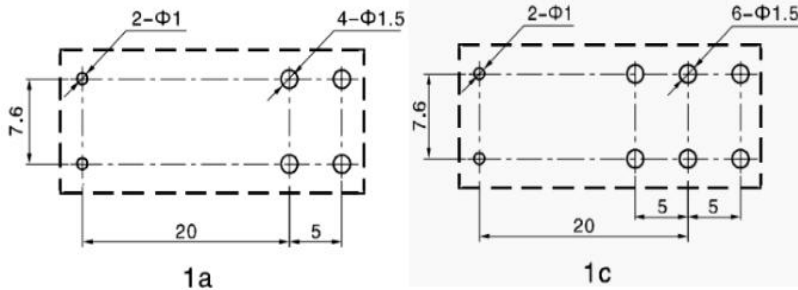
安装孔尺寸图 (底视图)
