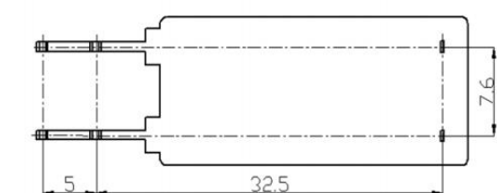
立式快接端子
