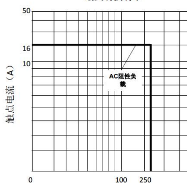
触点电压 (V)
