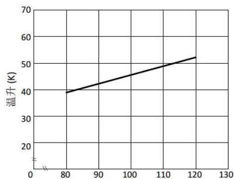
线圈额定电压百分比
