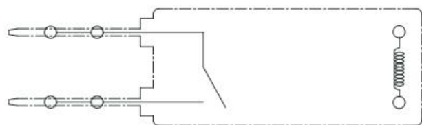
1A 接线图 (底视图)
