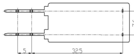
卧式快接端子
