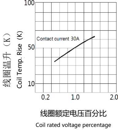
线圈温升 Coil Temp. Rise
