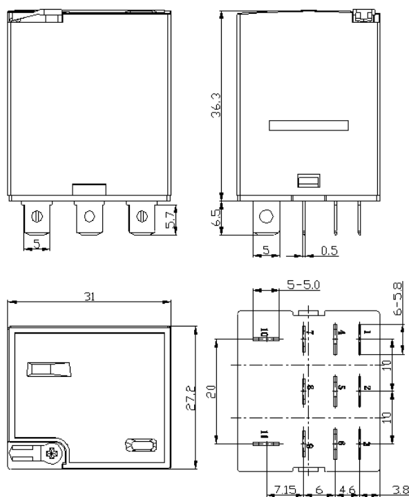
旋转型插座式 Rotary socket type
