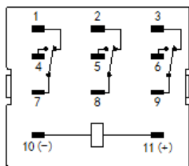
C 型 C type
