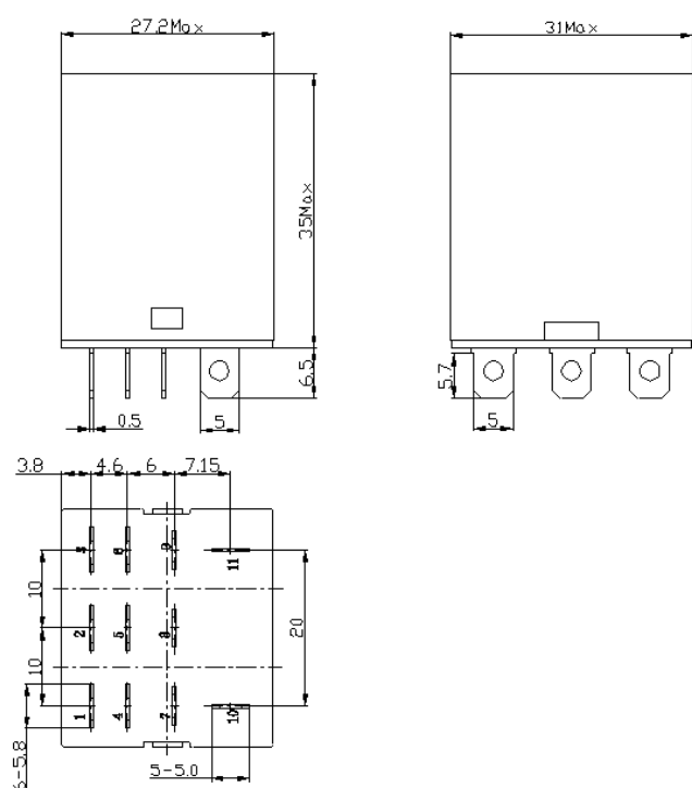
普通型插座式: General type socket type
