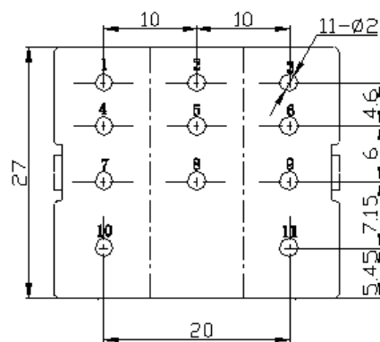
安装尺寸 (底视) :PCB 型 Mounting size (bottom view) : PCB type
