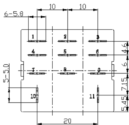
安装尺寸 (底视) :插座型 Mounting size (bottom view) : Socket type
