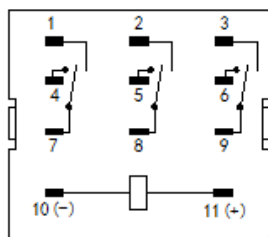
A 型 A type
