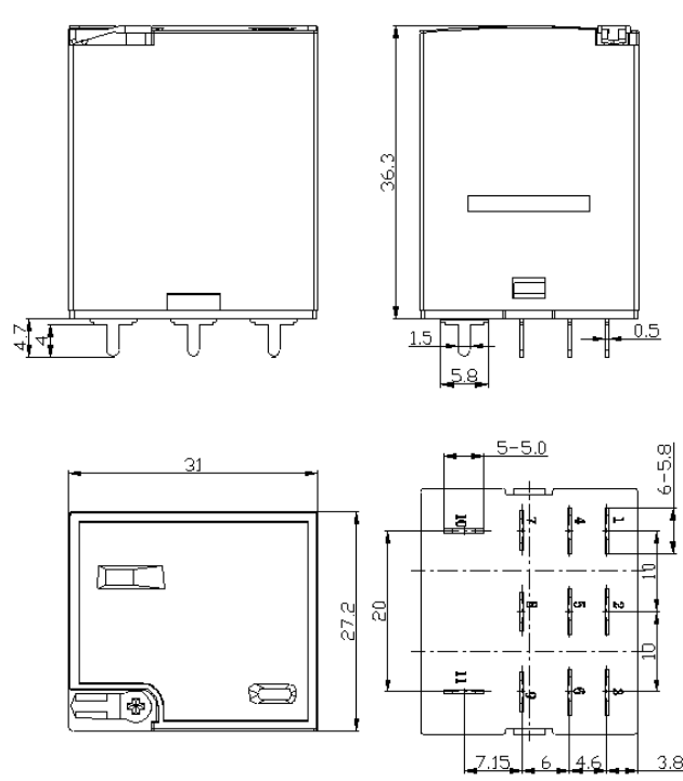
旋转型 PCB 式 Rotary PCB type
