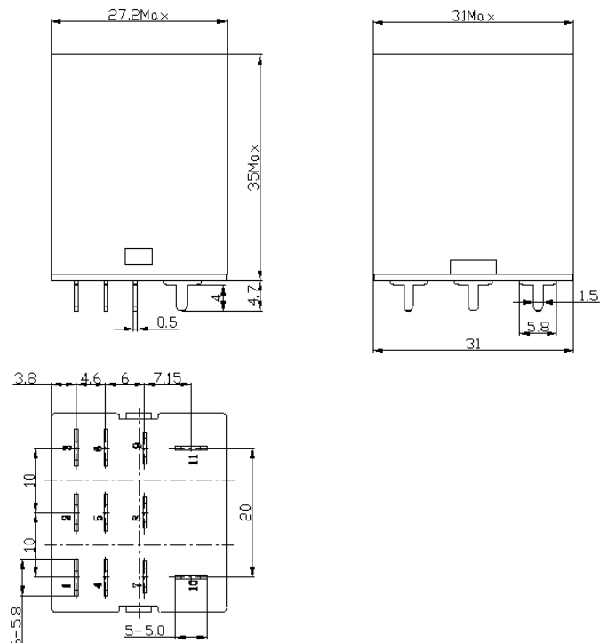
普通型 PCB 式 General purpose PCB type
