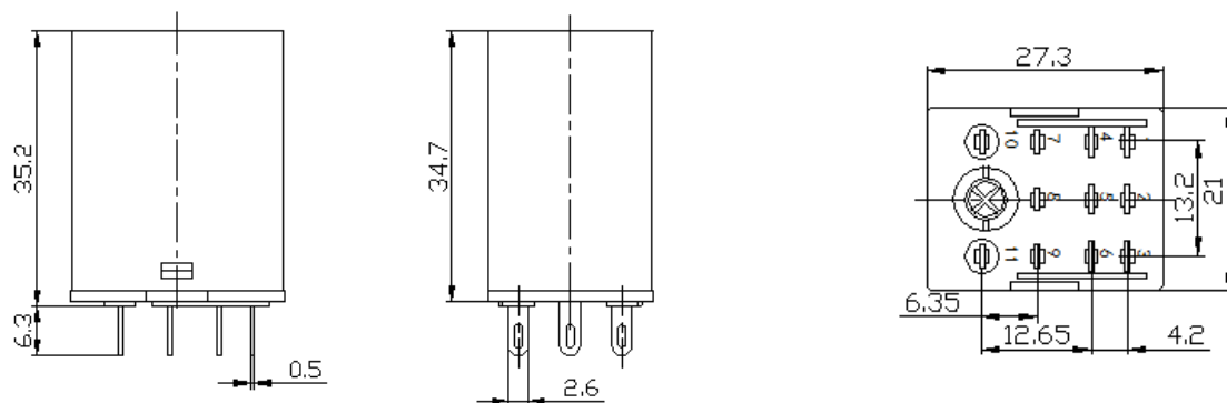
普通型插座式 General type socket type
