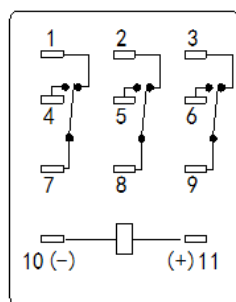
C 型 C type
