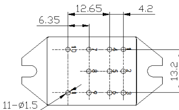
安装尺寸 (底视): 法兰型 Mounting size (bottom view): Flange type
