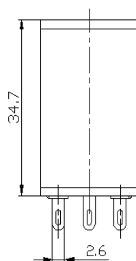
法兰型插座式 Flange socket type
