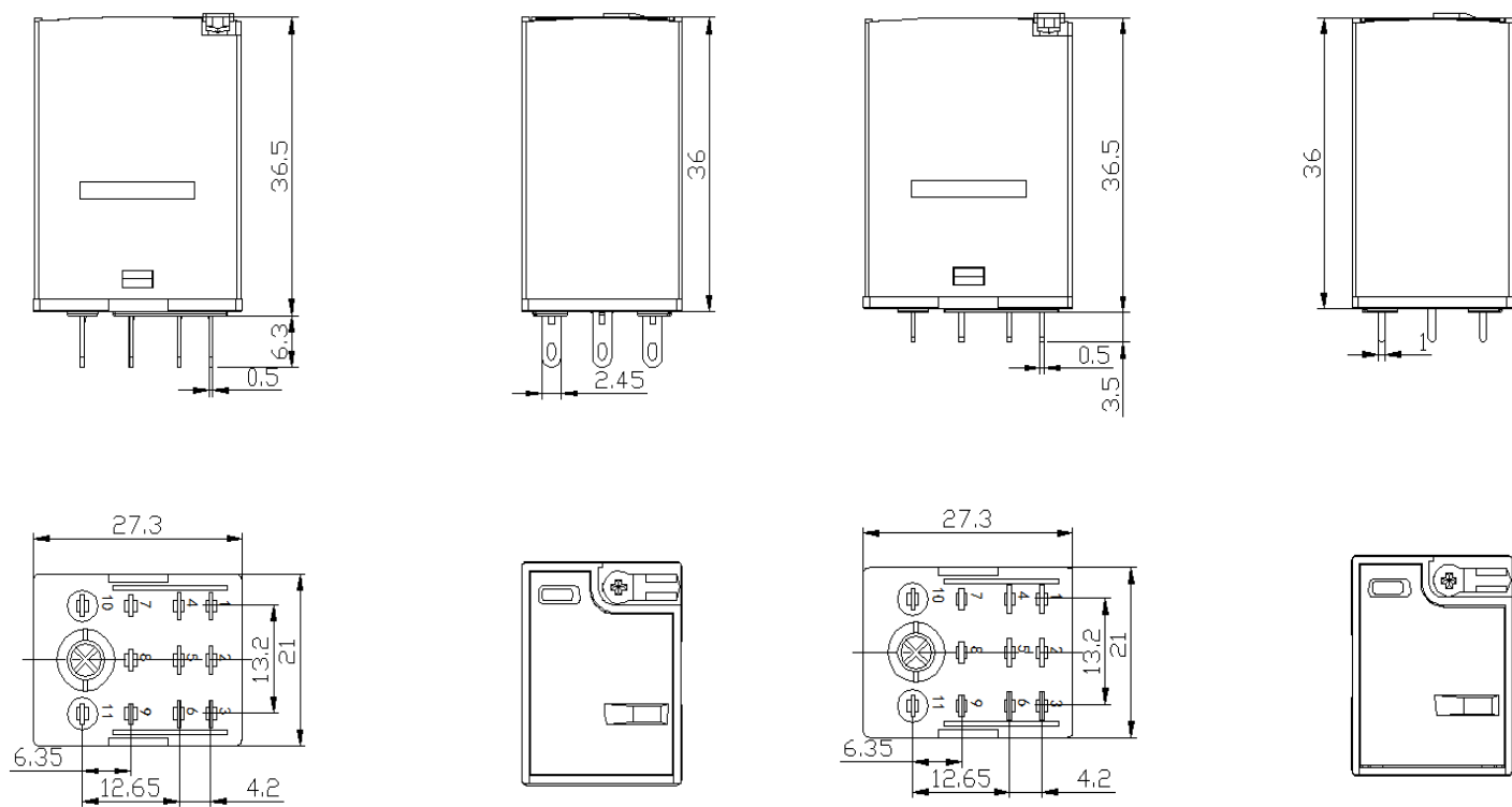
旋转型插座式 Rotary socket type
