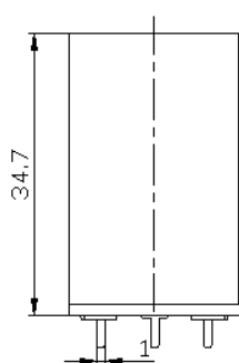
普通型 PCB 式 General purpose PCB type
