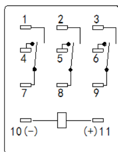
A 型 A type
