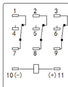
B 型 B type
